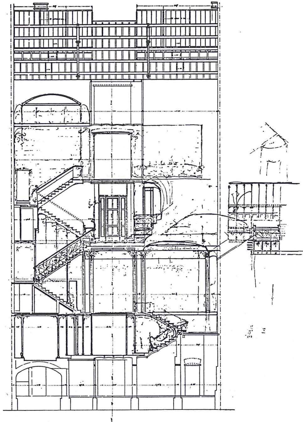
Hôtel Solvay. Coupe transversale (Archives Jean Delhaye)
