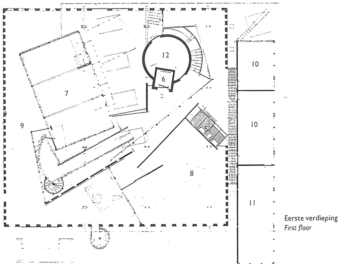
bibliotheek Zeewolde (1985-1989)
