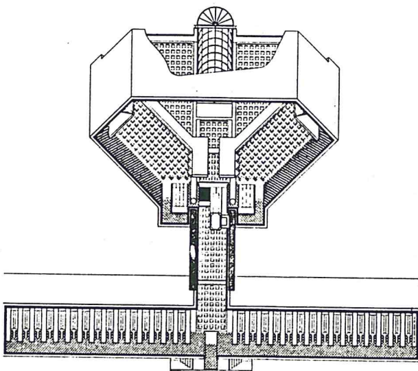
Banca del Gottardo a Lugano Library of the Convento dei Cappuccini Interior view: the reading room Axonometric
